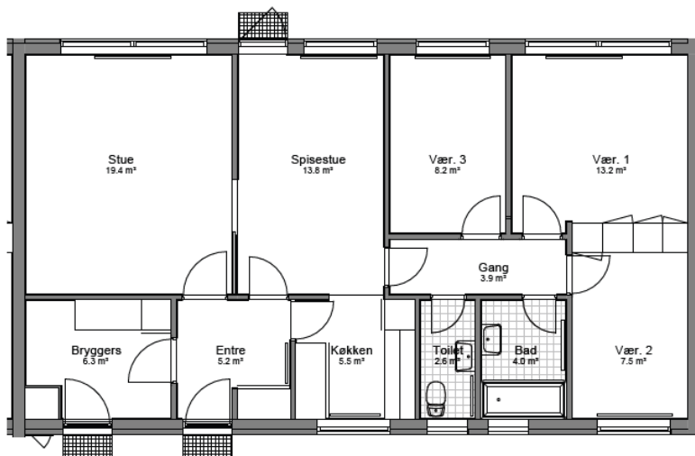
EKSISTERENDE FORHOLD 106 M 2 5-VÆRELSES BOLIG
